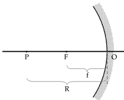
Gambar 17.7 Cermin cekung
