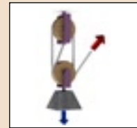
Katrol ganda dengan tarikan ke atas, KM = 3 (jumlah tali)
